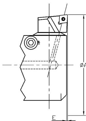
ABB. 2 FORM RHOMBISCH WENDEPLATTEN
