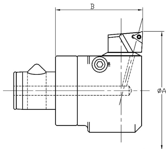
ABB. 1 FORM DREIKANT WENDEPLATTEN
