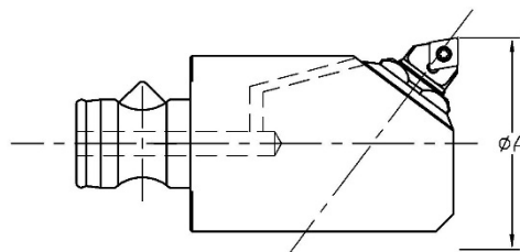
ABB. 2 FORM RHOMBISCH WENDEPLATTEN
