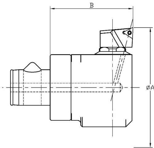
ABB. 1 FORM DREIKANT WENDEPLATTEN
