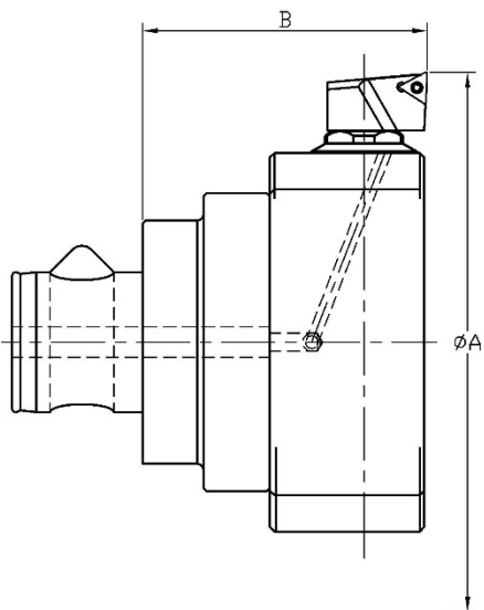
ABB. 1 FORM DREIKANT WENDEPLATTEN
