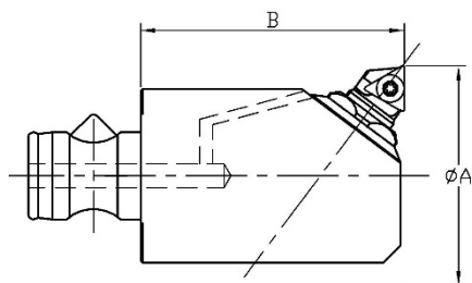
ABB. 1 FORM DREIKANT WENDEPLATTEN
