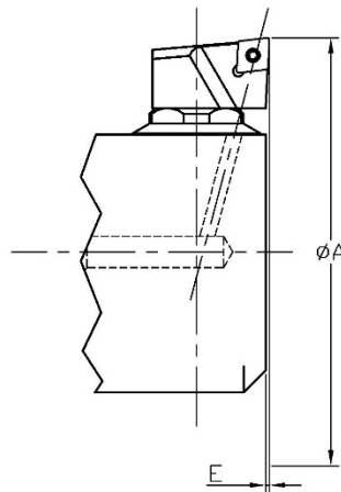
ABB. 2 FORM RHOMBISCH WENDEPLATTEN
