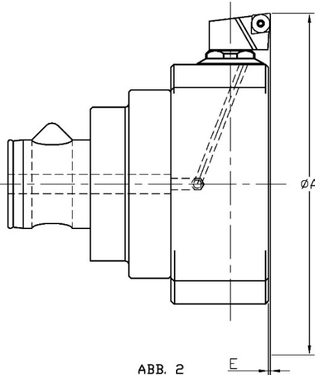
ABB. 2 FORM RHOMBISCH WENDEPLATTEN
