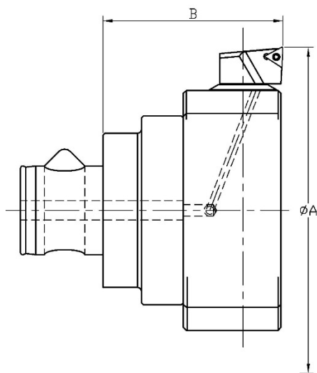
ABB. 1 FORM DREIKANT WENDEPLATTEN
